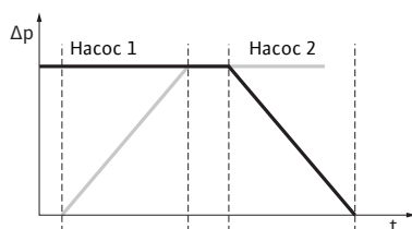
Fig.21: Смена насоса
