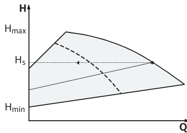
Fig.20: Регулирование \Delta p -v (работа двух насосов)
