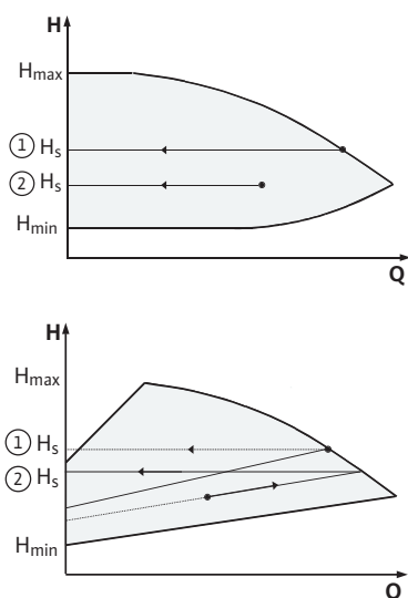
Fig. 47: Регулирование Δp-с/Δp-v
