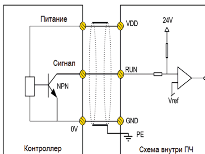
Подключение дискретных входов в режиме PNP
