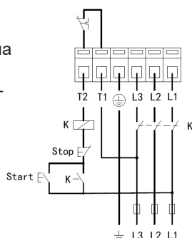
Рис. 3.2 Схема подключения с нейтральным проводом
