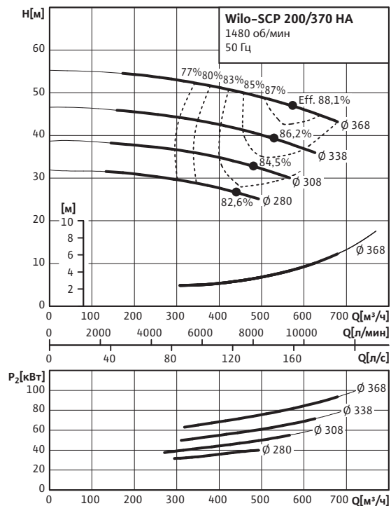
Wilo-SCP 200/370 HA
