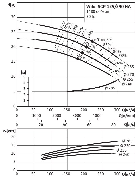
Wilo-SCP 125/290 HA
