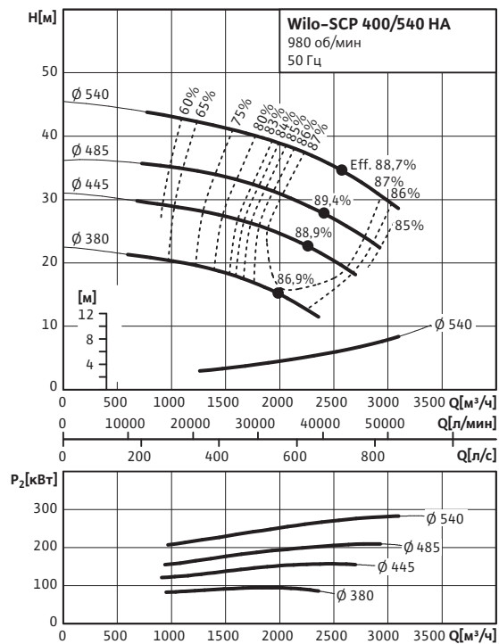
Wilo-SCP 400/540 HA
