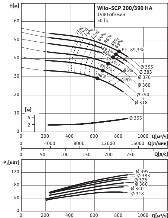
Wilo-SCP 200/390 HA
