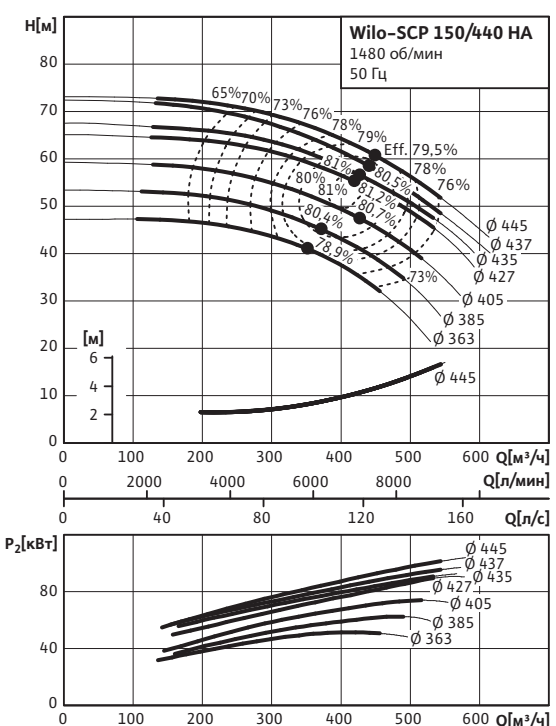
Wilo-SCP 150/440 HA
