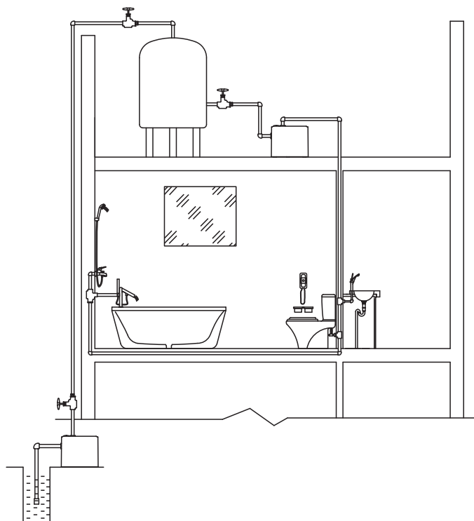
Забор воды из колодца и повышение давления в системе водоснабжения
