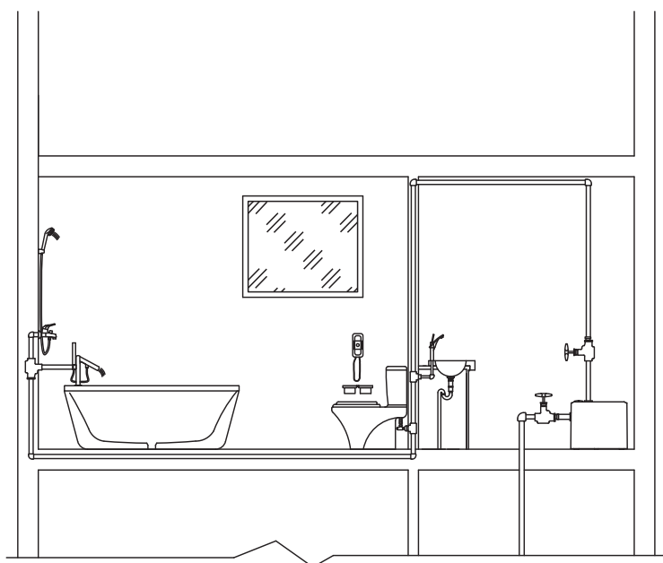
Повышение давления в системе водоснабжения
