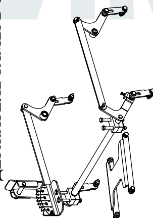
ДЕРЖАТЕЛЬ РАМЫ В СБОРЕ
