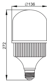
Рисунок 31 – Лампа LED-HP, 80 Вт, цоколь E40
