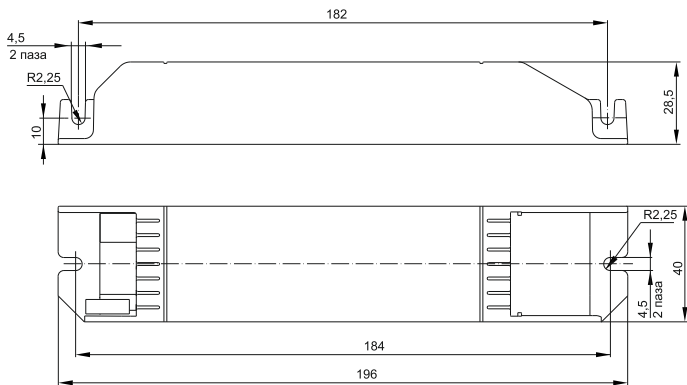
Рисунок 1 – Конвертер БАП40-1,0(3,0); БАП80-1,0(3,0)
