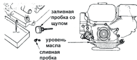
Рисунок 9 - Замена масла в двигателе
