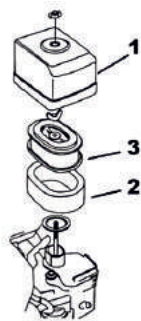
Рисунок 8 – Воздушный фильтр
