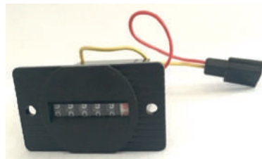
Рисунок 6 – Счетчик моточасов
