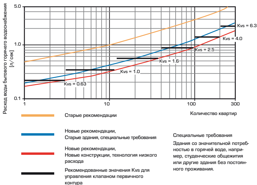
ТЕХНИЧЕСКИЕ УСЛОВИЯ - БЫТОВАЯ СИСТЕМА ГОРЯЧЕГО ВОДОСНАБЖЕНИЯ, ПЕРВИЧНЫЙ КЛАПАН В РАЙОННОМ ТЕПЛОПУНКТЕ
