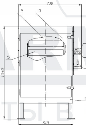
Рис. 1 - Габаритные размеры и схематическое устройство электропечи.
