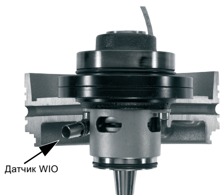
Рис. 16 Аналоговый датчик воды в масле
