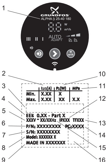
Рис. 2 Фирменная табличка
