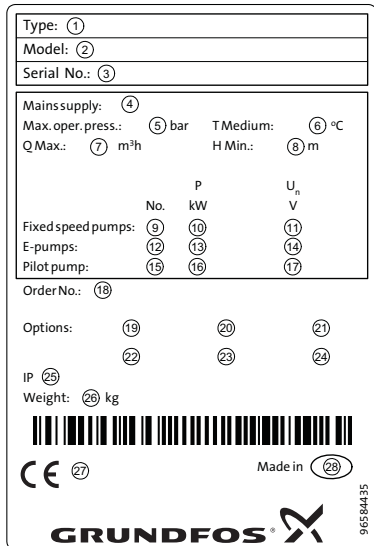
Рис. 1 Заводская табличка, установка повышения давления
