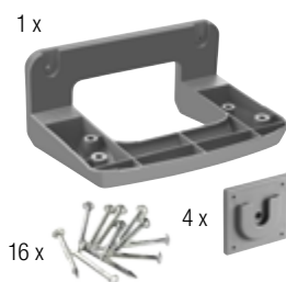
Кронштейн для горизонтального модуля
