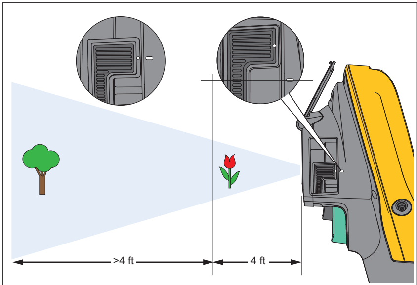
Рис. 2. IR-OptiFlex Focus
