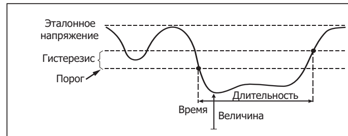
Рисунке 8. Характеристики кратковременного понижения напряжения
