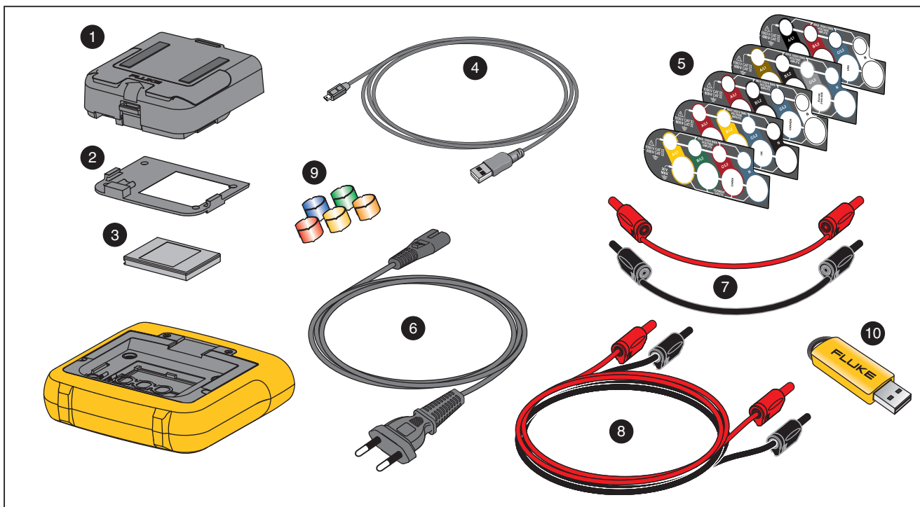
Рисунке 11. Заменяемые компоненты
