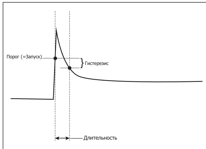
Рисунке 10. Пусковые характеристики и отношение к меню запуска
