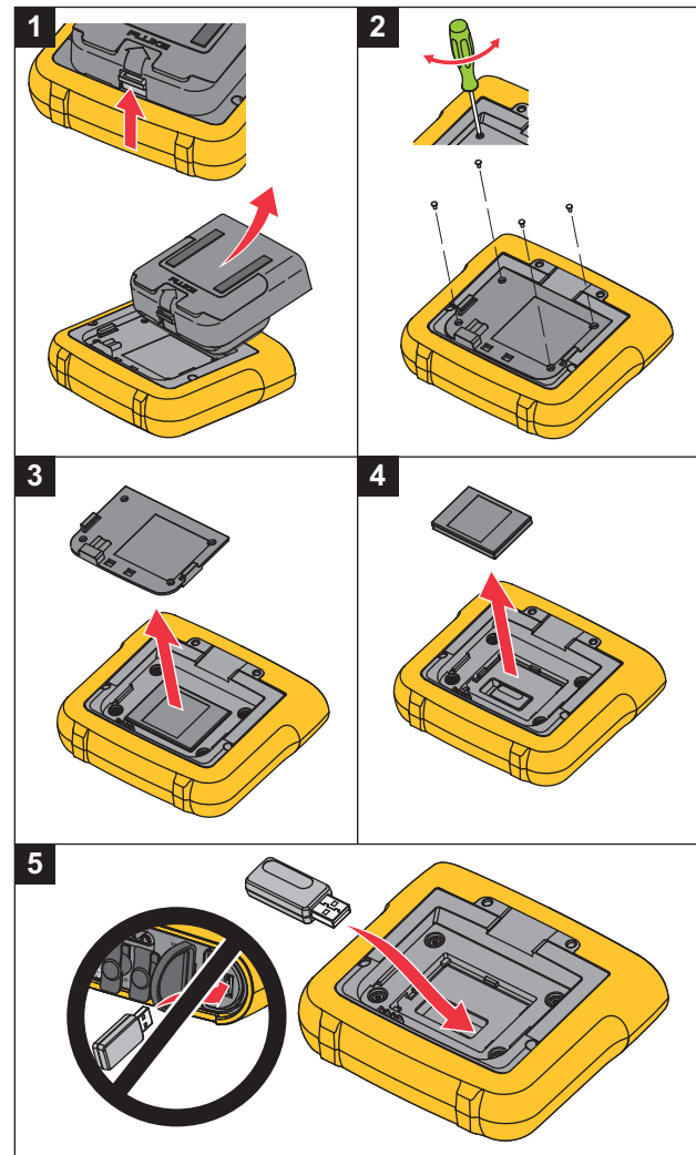
Рисунке 1. Установка переходника
