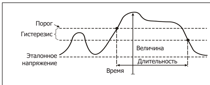
Рисунке 7. Характеристики кратковременного повышения напряжения
