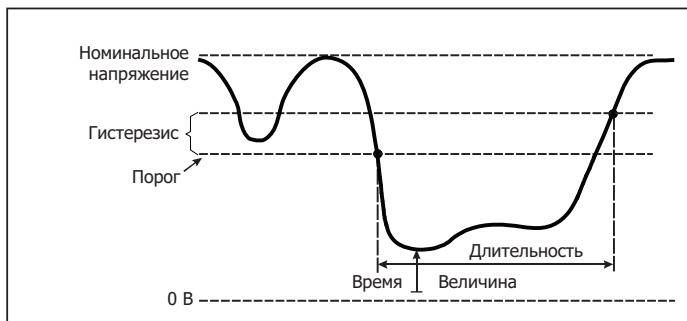
Рисунке 9. Характеристики прерывания напряжения
