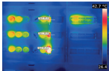
Нагрузка в блоках предохранителей распределяется неравномерно
