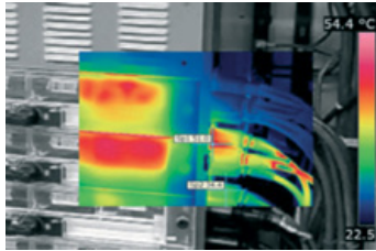
Перегревающийся разъем
