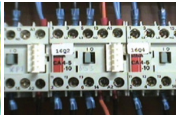
Горячая точка указывает на короткое замыкание, которое может стать причиной пожара
