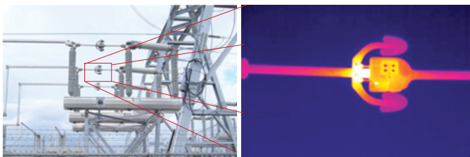
Тепловизионные камеры позволяют проверять высоковольтное оборудование с безопасного расстояния, обеспечивая безопасность персонала
