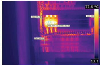
Предохранители, которые видны на ИК-изображении, перегружены и требуют замены
