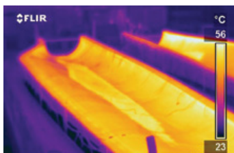
ИК-изображение пресс-формы
