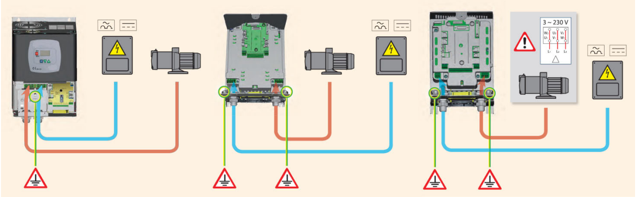
Şekil 6: Elektrik bağlantıları
