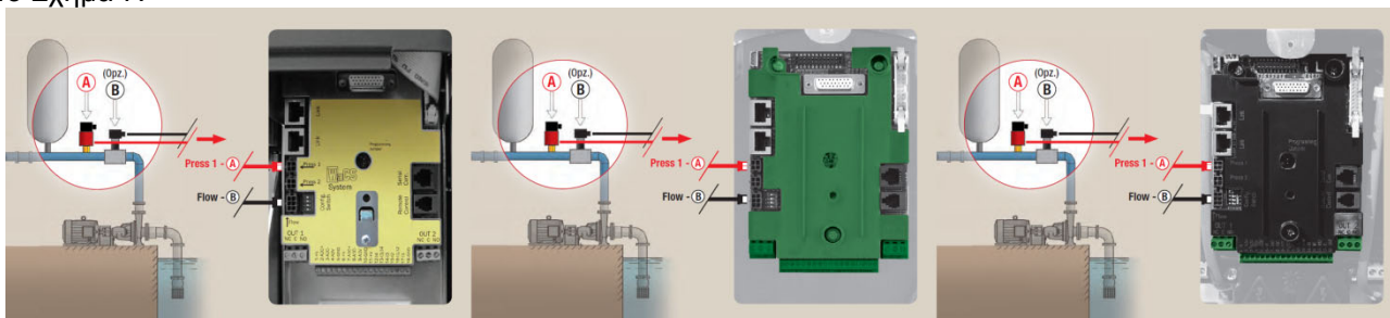
Σχήμα 9: Συνδέσεις αισθητήρων
