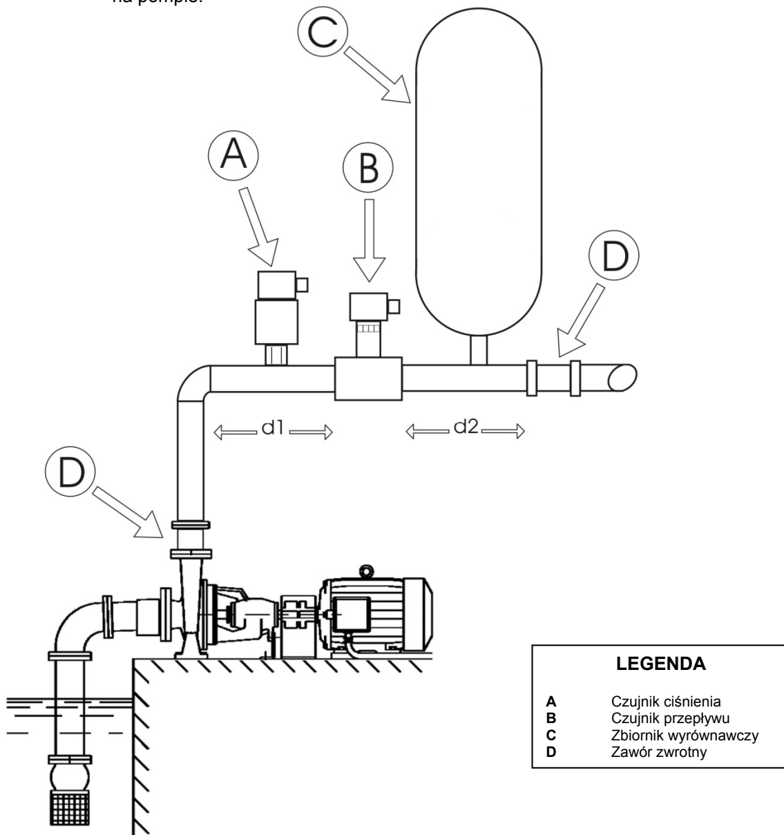
Rys. 8: Instalacja hydrauliczna
