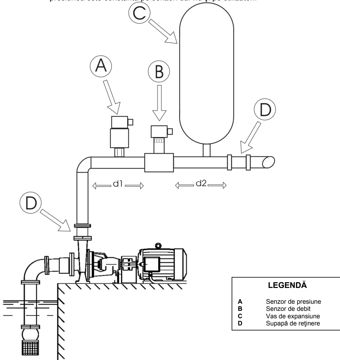
Figura 8: Instalația hidraulică
