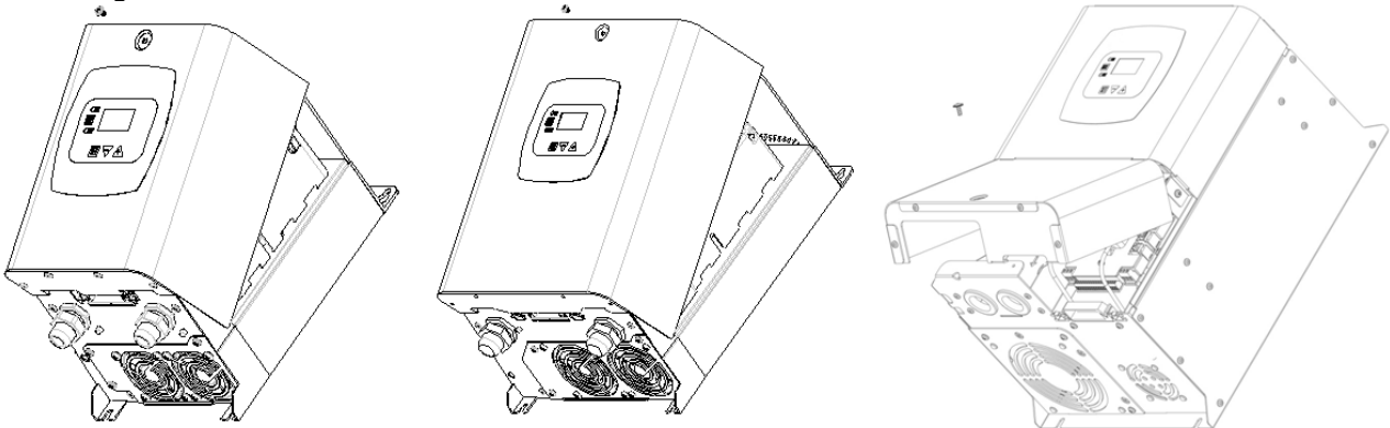
Abbildung 3: Ausbauen des Deckels für den Zugriff auf die Anschlüsse
