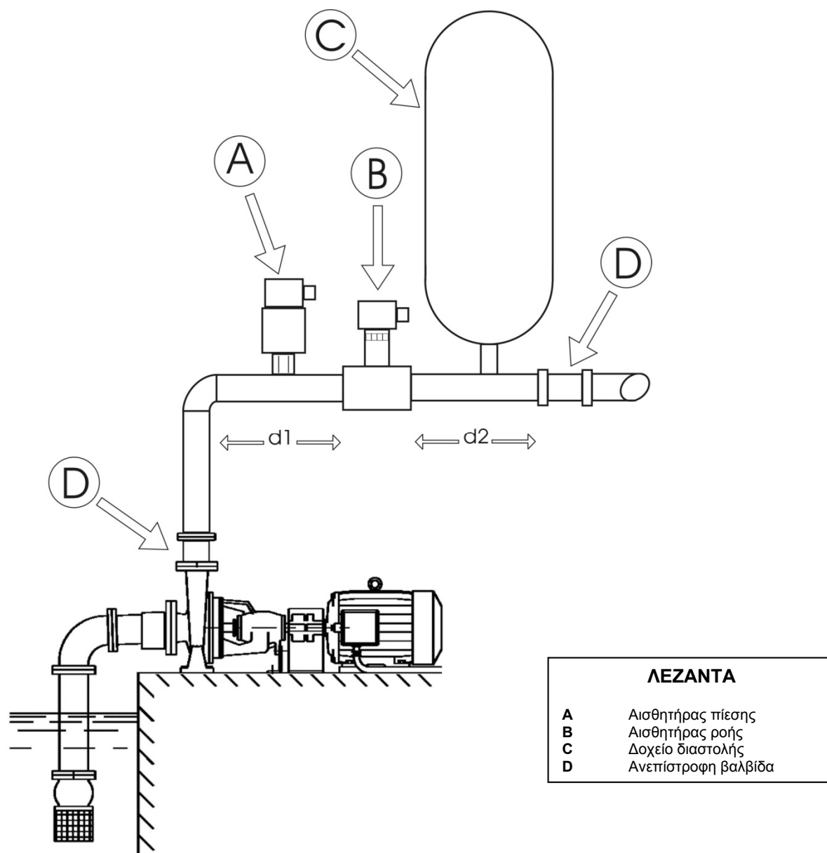
Σχήμα 8: Υδραυλική εγκατάσταση
