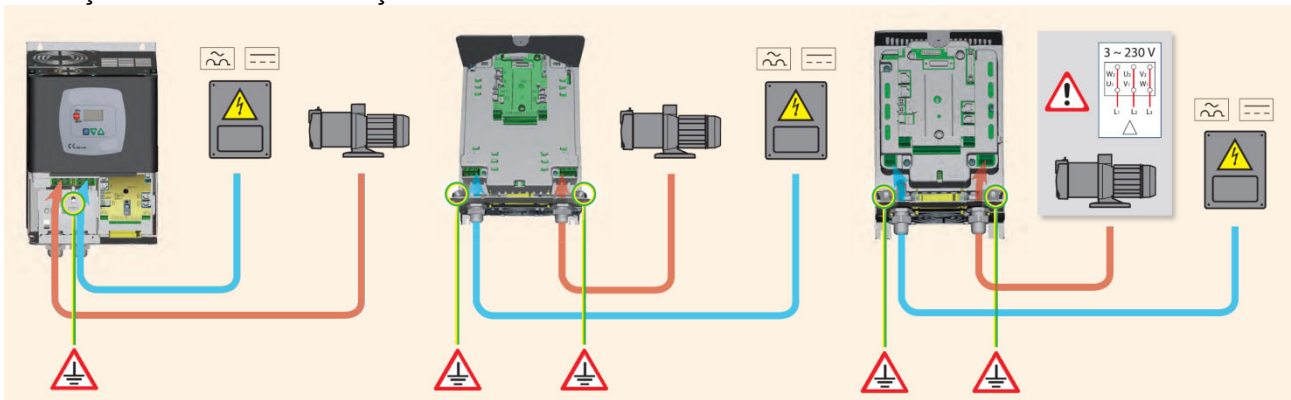
Figura 6: Conectări electrice
