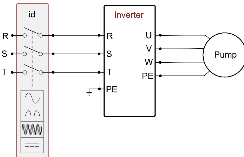
Fig. 5b: Exempel på installation med trefasmatning
