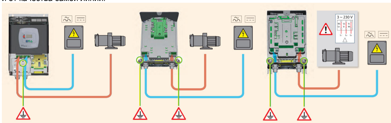
Рисунок 6: Электрические соединения
