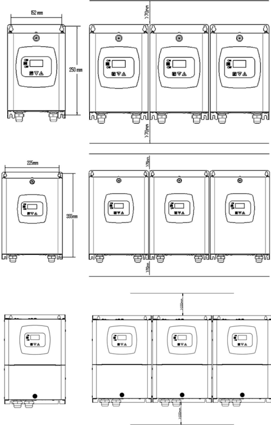
Şekil 2: Hava sirkülasyonu tesiatı ve minimum açıklık
