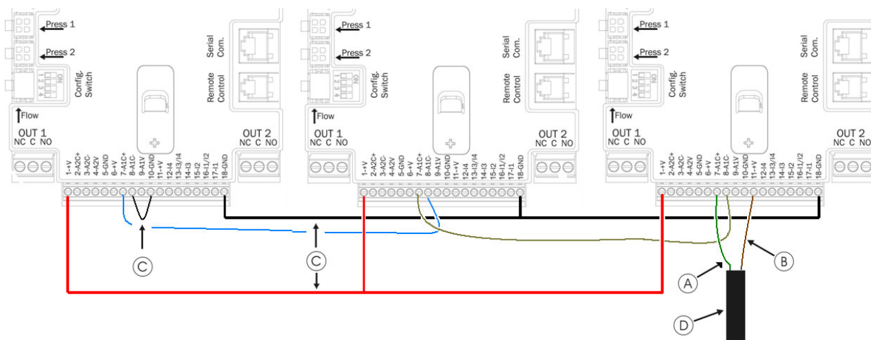
Σχήμα 11: Σύνδεση αισθητήρα πίεσης 4 – 20 mA σε ένα σύστημα multi invertir
