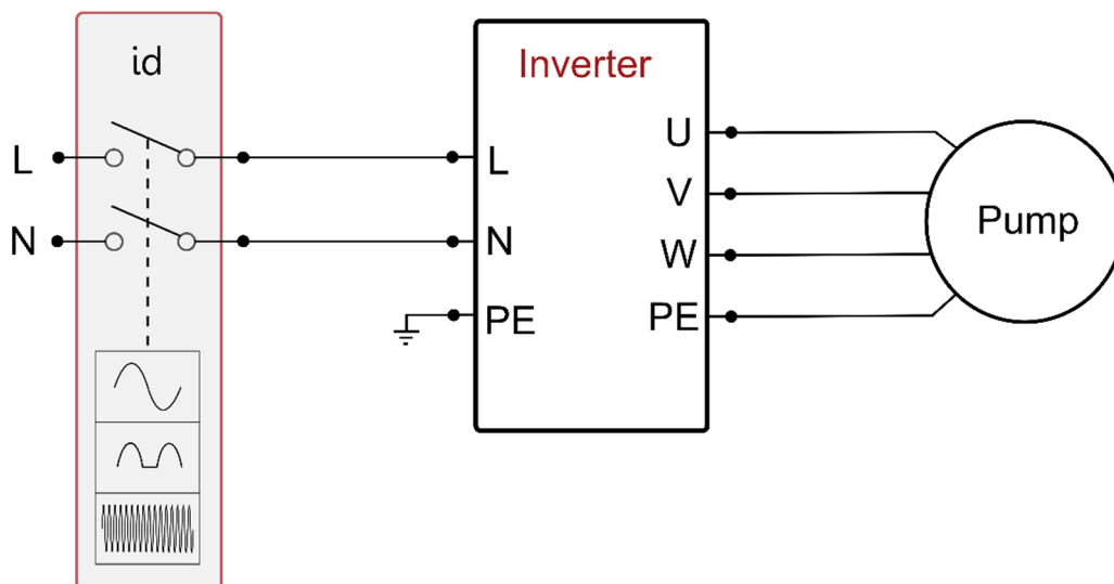
Fig. 4a: Exempel på installation med enfasmatning
