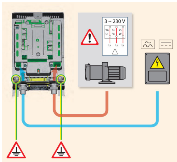
Фигура 7: Съвързване на помпа AD 2.2 AC - 1.5 AC - 1.0 AC
