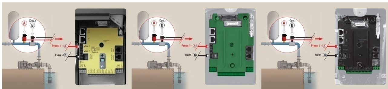
Obrázek 9: Připojení snímačů
