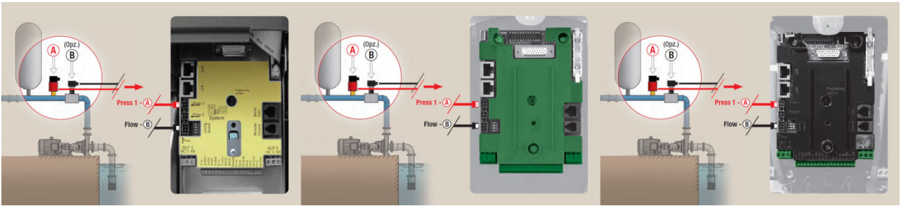
Figura 9: Conexiones de los sensores
