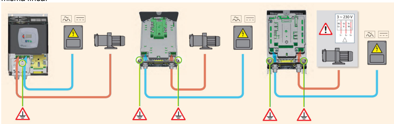
Figura 6: Conexiones eléctricas
