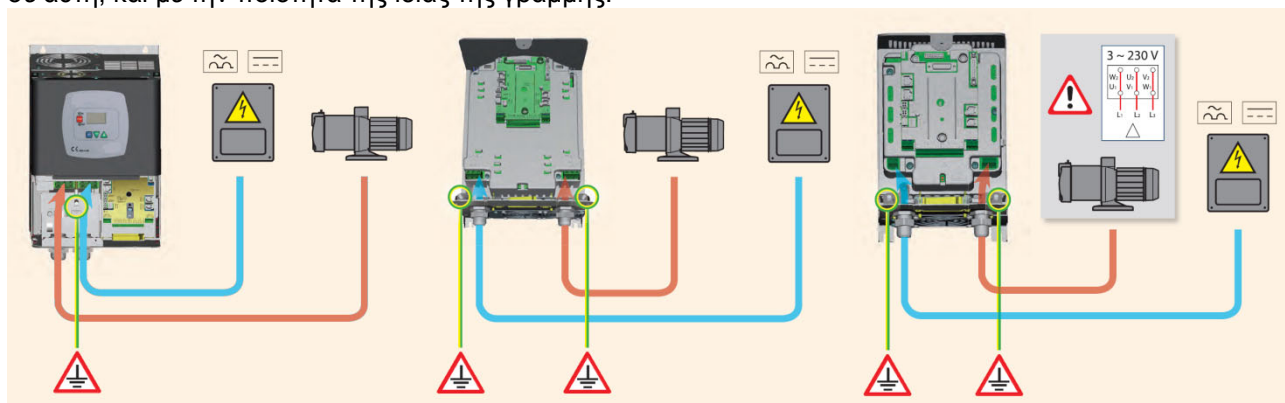
Σχήμα 6: Ηλεκτρολογικές συνδέσεις
