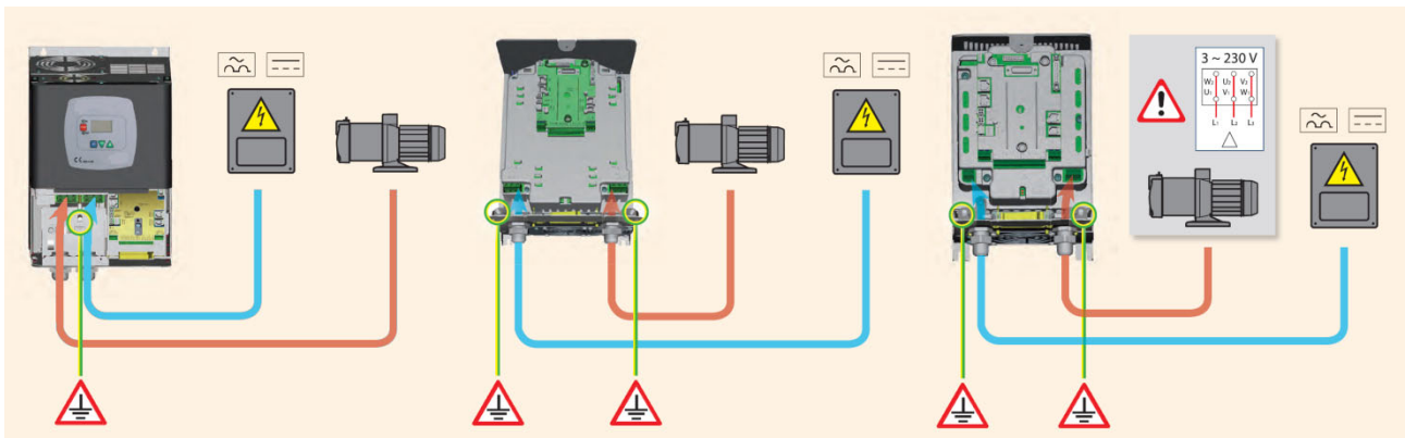
Figure 6: Connexions électriques
