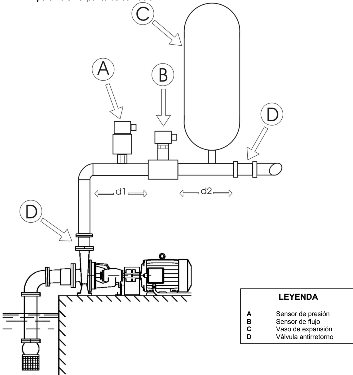
Figura 8: Instalación hidráulica
