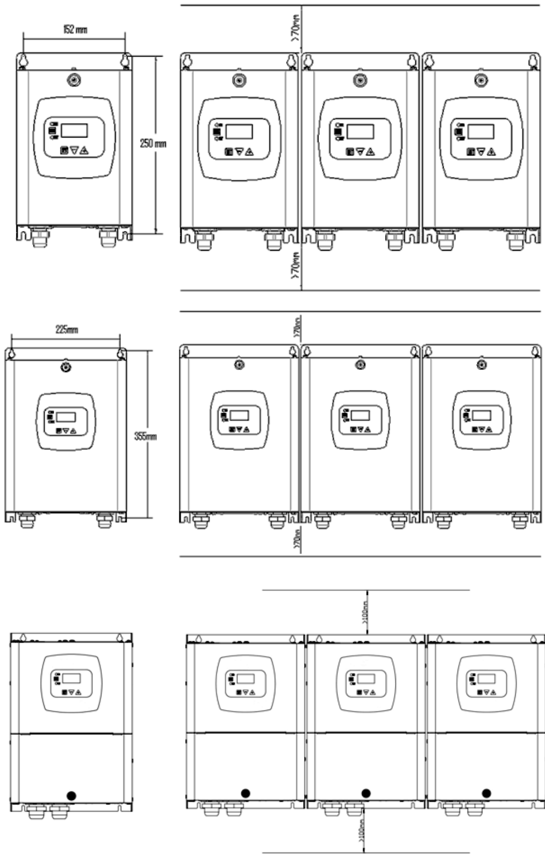
Fig. 2: Fastsättning och min. utrymme för luftcirkulation
