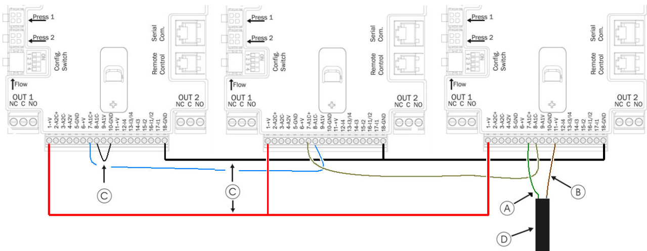
Fig. 11: Anslutning av trycksensor 4 - 20 mA i ett system med flera invertrar
