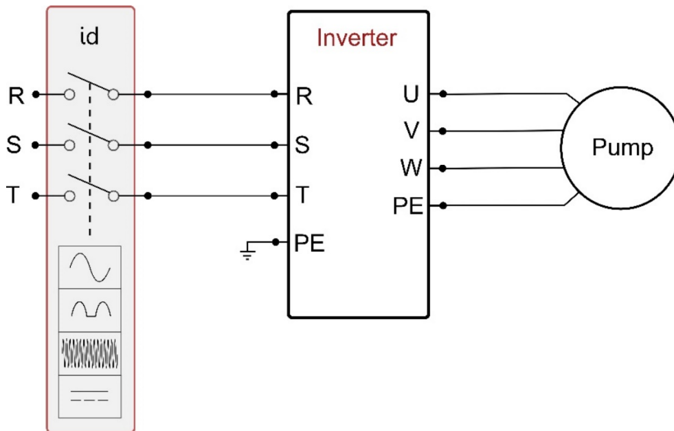
Figura 5b: Ejemplo de instalación con alimentación monofásica
