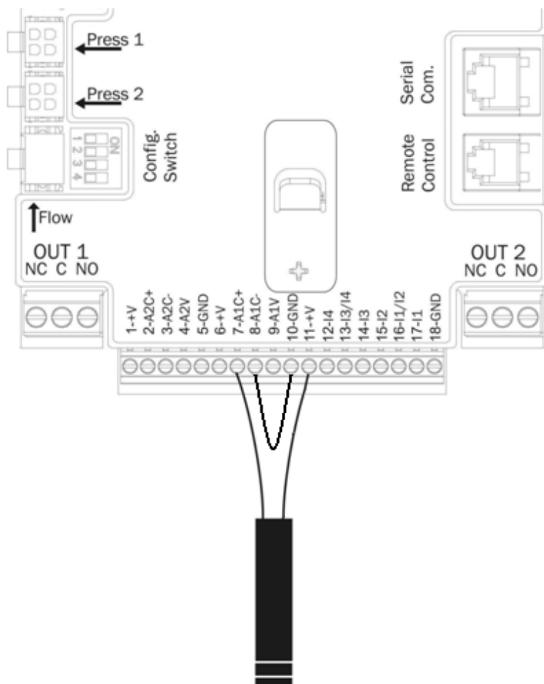
Фигура 10: Свързване на датчик за налягане по ток 4 - 20 мА
