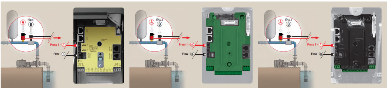
Figure 9: Connexions capteurs
