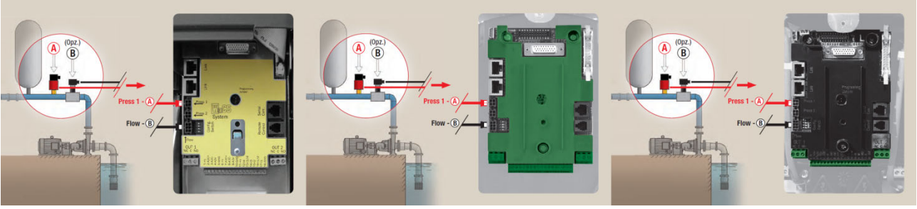
Şekil 9: Sensör bağlantıları
