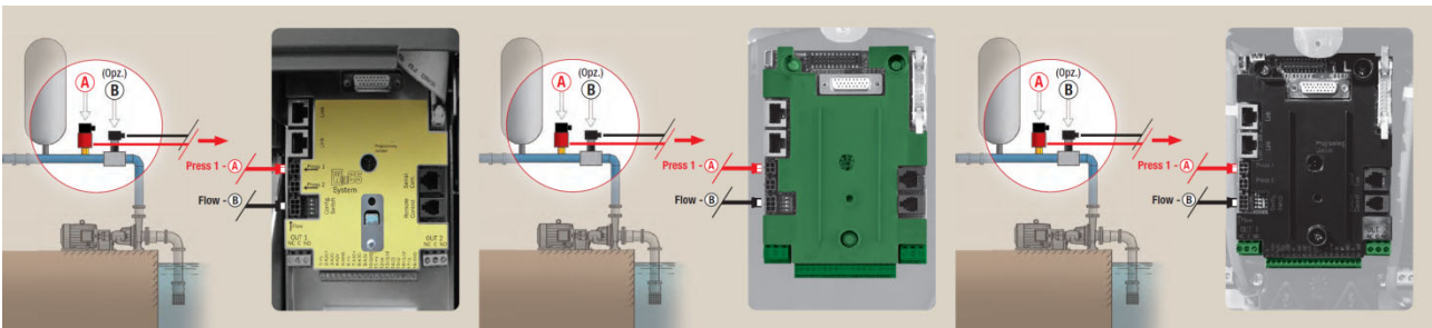
Afbeelding 9: Aansluitingen sensoren
