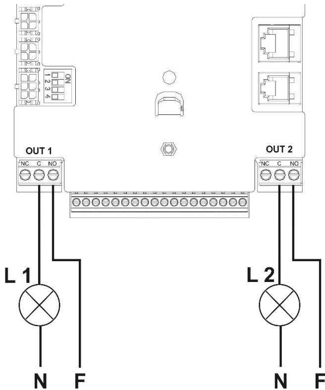
Figura 12: Exemplu de conectare a ieșirilor
