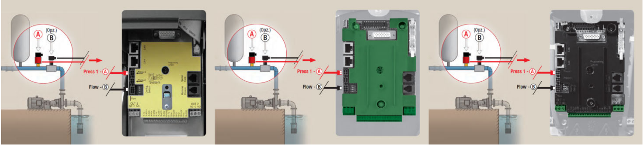
Figura 9: Conexiuni senzori
