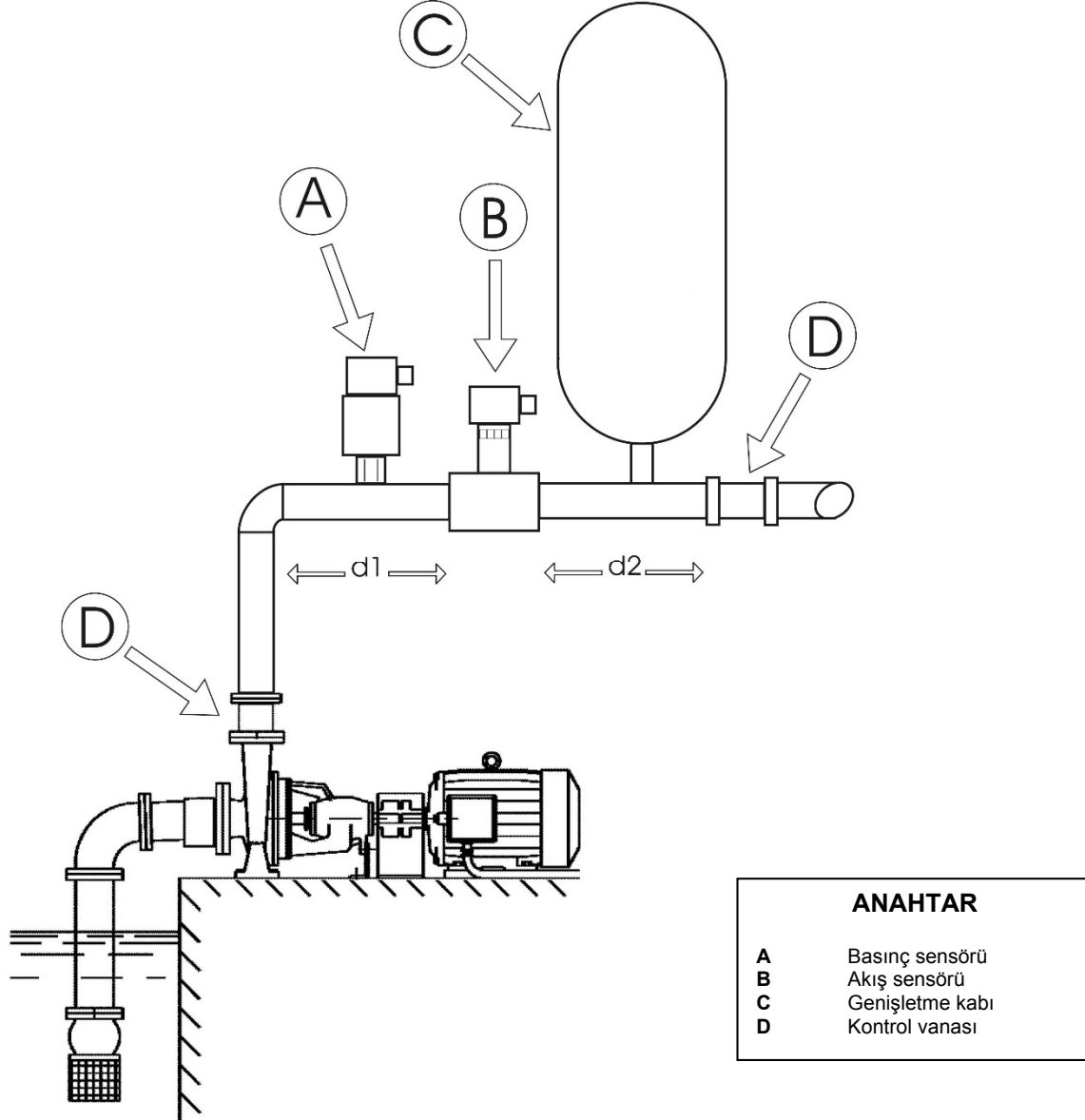
Şekil 8: Hidrolik kurulum
