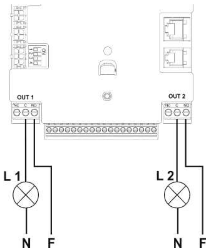
Fig. 11: Exempel på anslutning av utgångar
