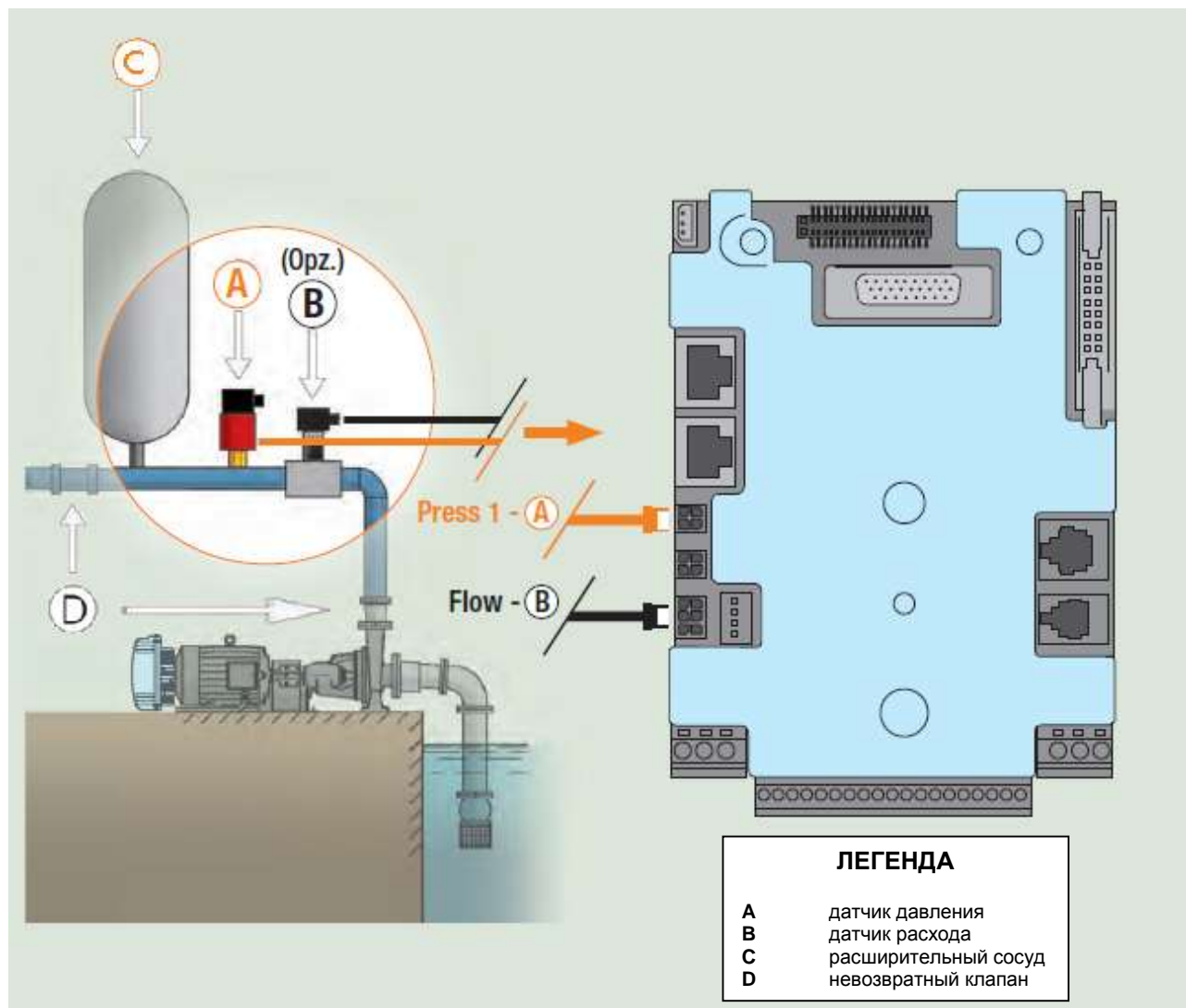
Рисунок 7: Гидравлический монтаж
