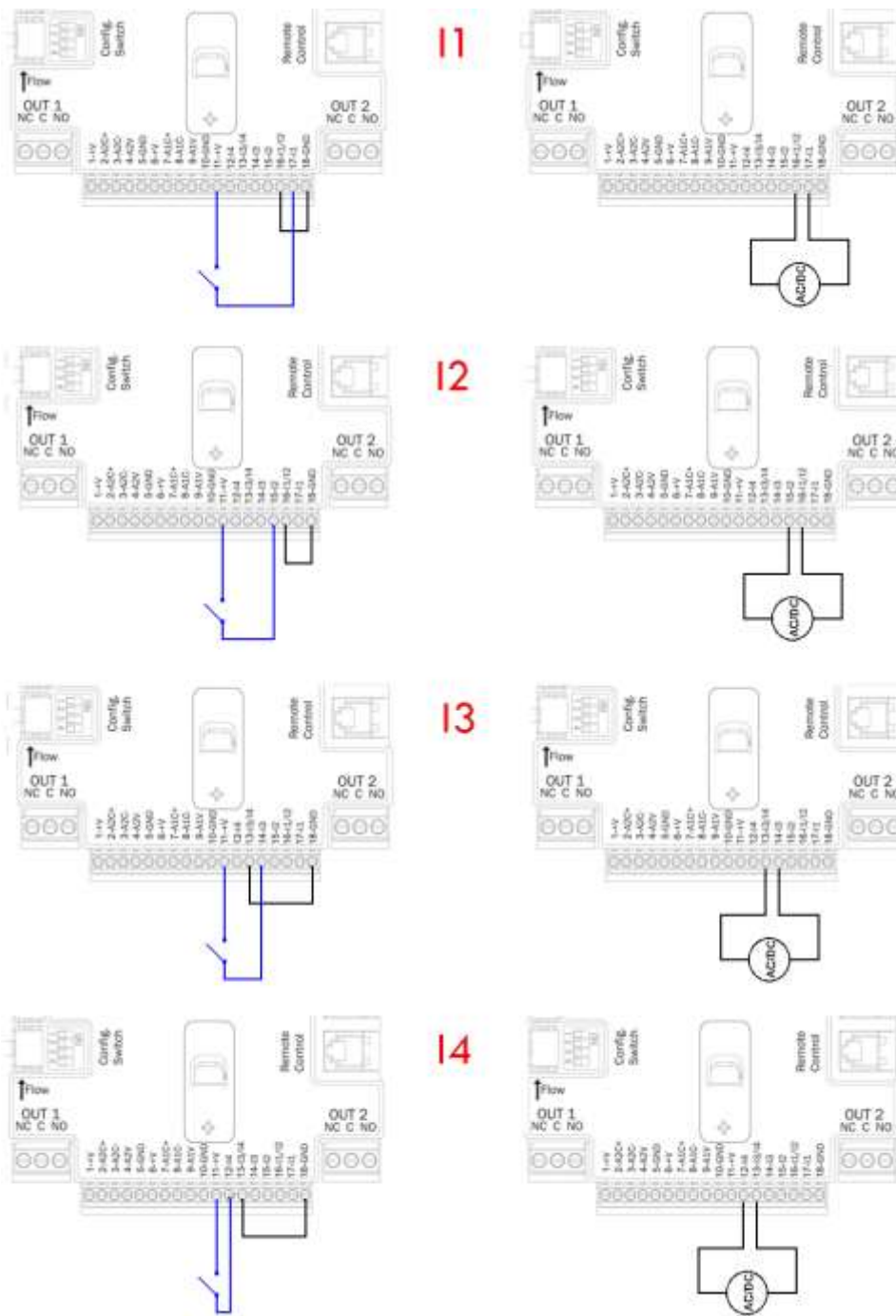
Kuva 12: Esimerkki tulojen liitännästä
