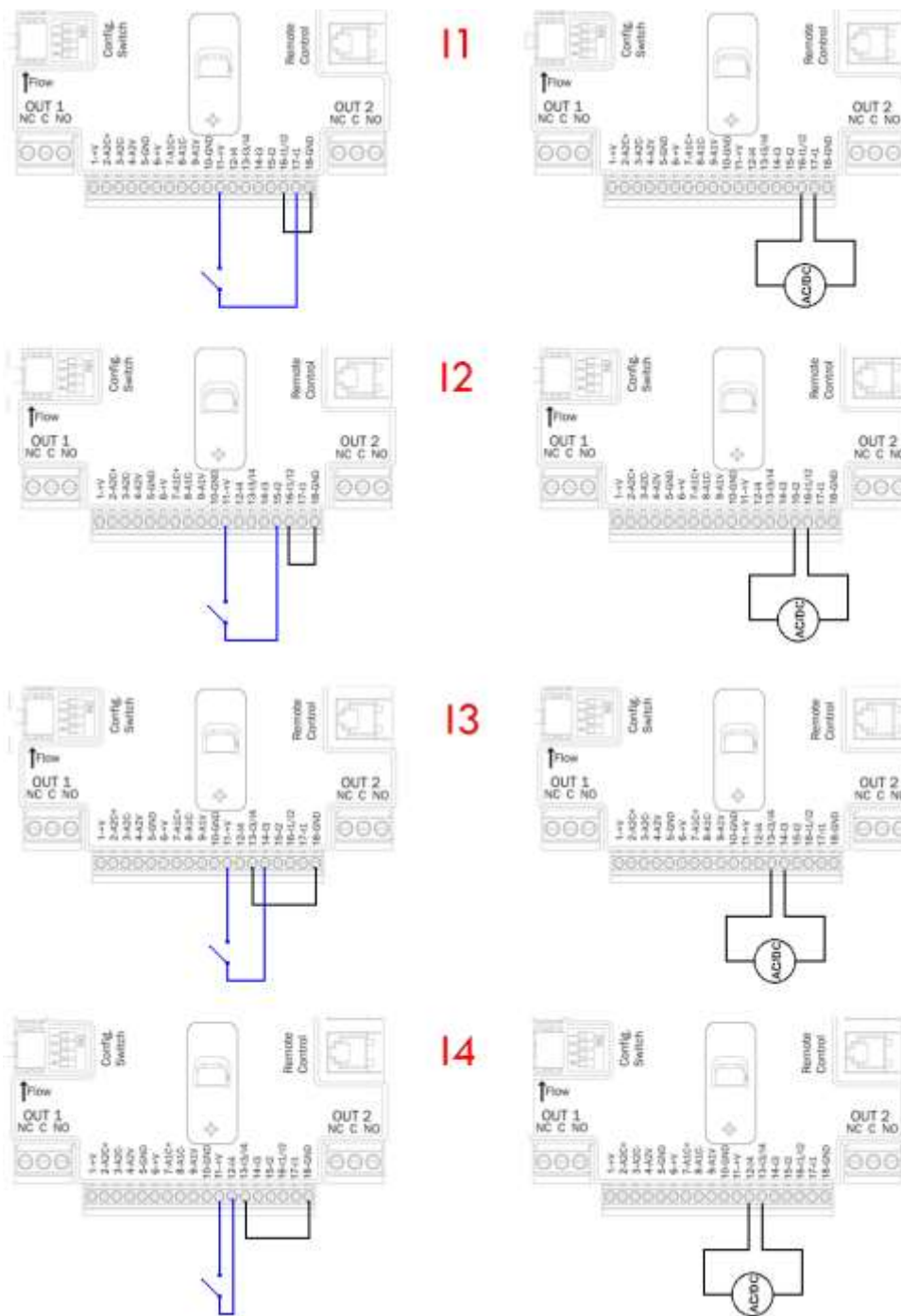
Фиг. 12: Пример на свързване на вход.
