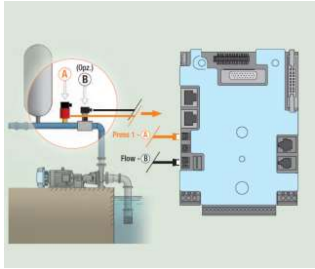
Şekil 8: Sensör bağlantıları
