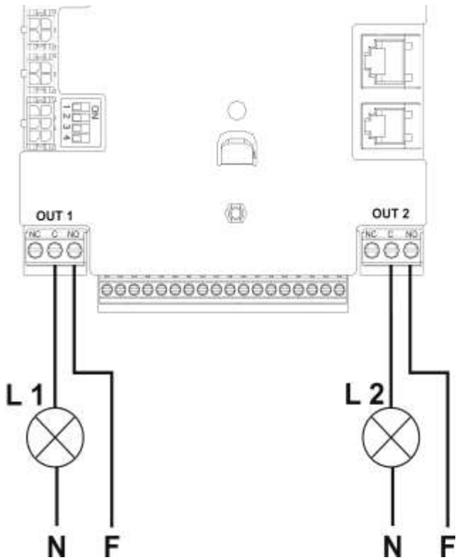
Figura 11: Ejemplo de conexión de las salidas
