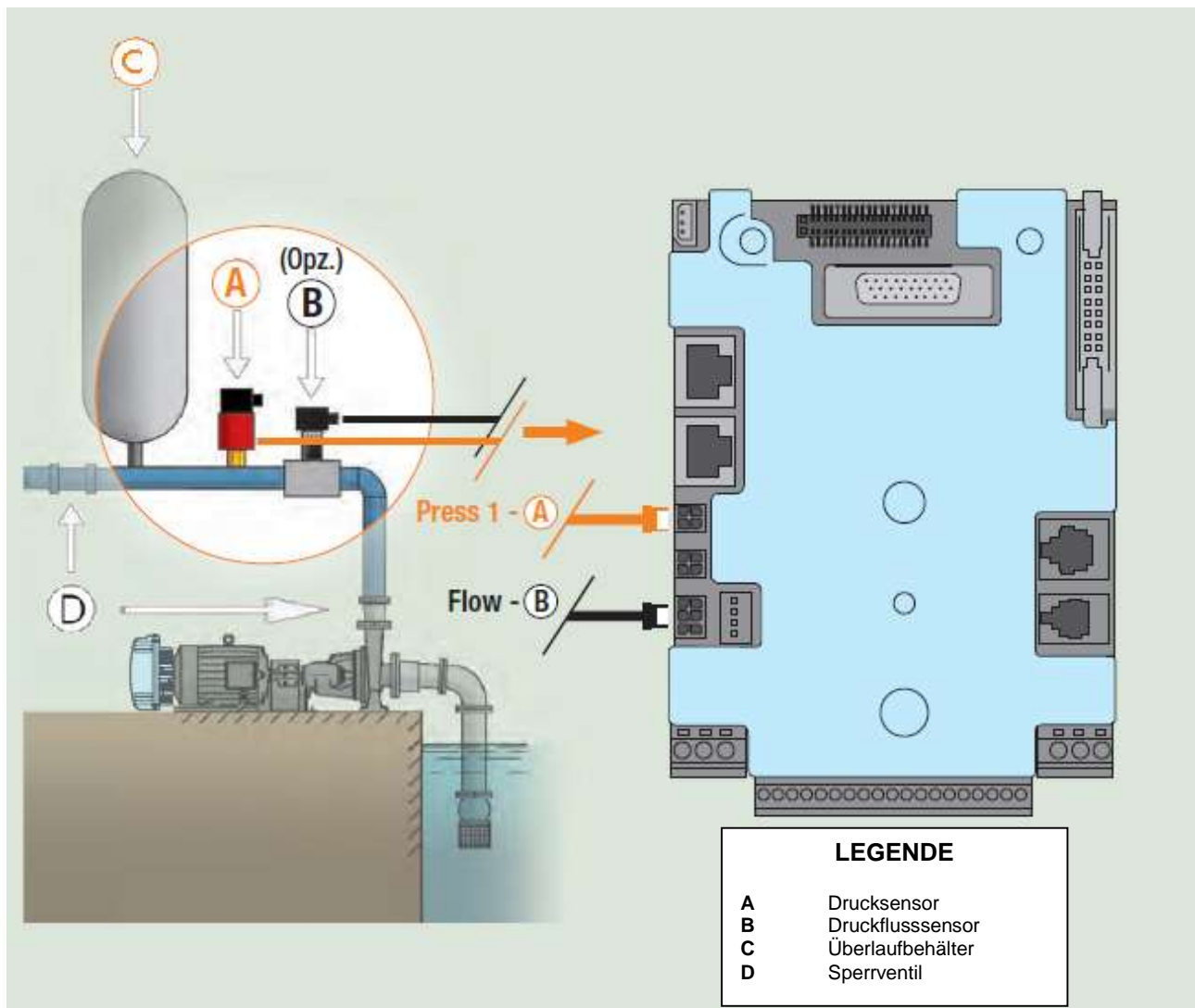
Abbildung 7: Hydraulik-Installation
