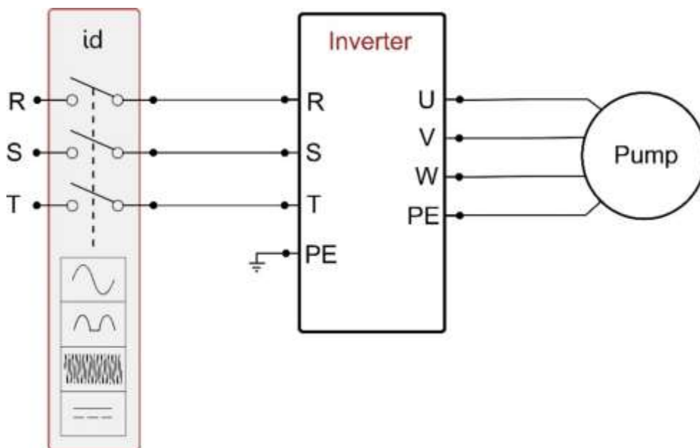
Kuva 4b: Asennusesimerkki kolmivaiheisella virtalähteellä
