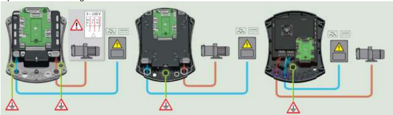
5.ábra: Elektromos bekötések
