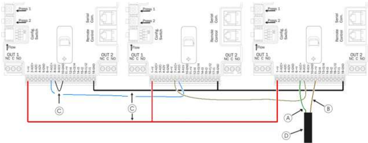
Фиг. 10: Свързване на 4 - 20 mA датчик за налягане в мултиинверторна верига
