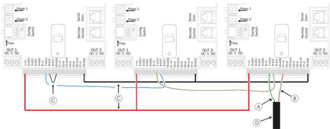
Kuva 10: Paineanturin liitäntä 4 - 20 mA multi-invertter-järjestelmässä
