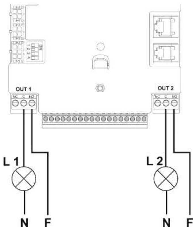
фиг. 11: Пример на свързване на изходите
