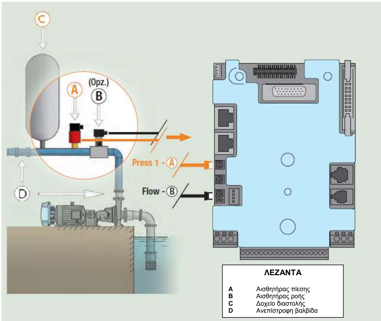
Σχήμα 7: Υδραυλική εγκατάσταση
