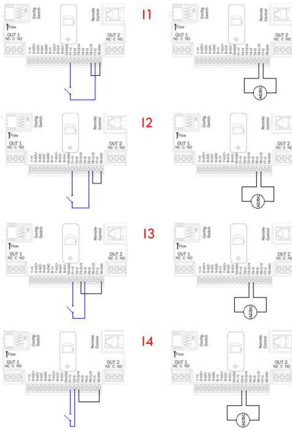
Obrázek 12: Příklad zapojení vstupu
