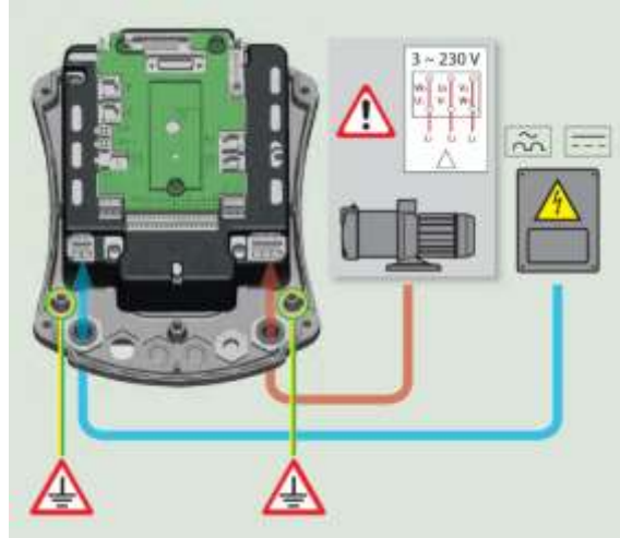
6.ábra: Szivattyú bekötés MCE 22/P – MCE 15/P – MCE 11/P
