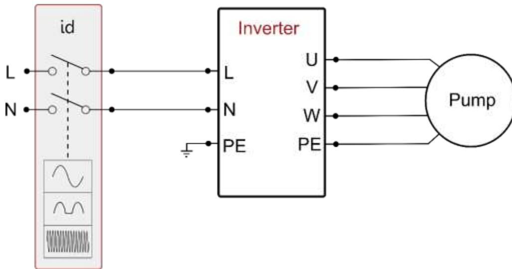
Kuva 3a: Asennusesimerkki yksivaiheisella virtalähteellä
