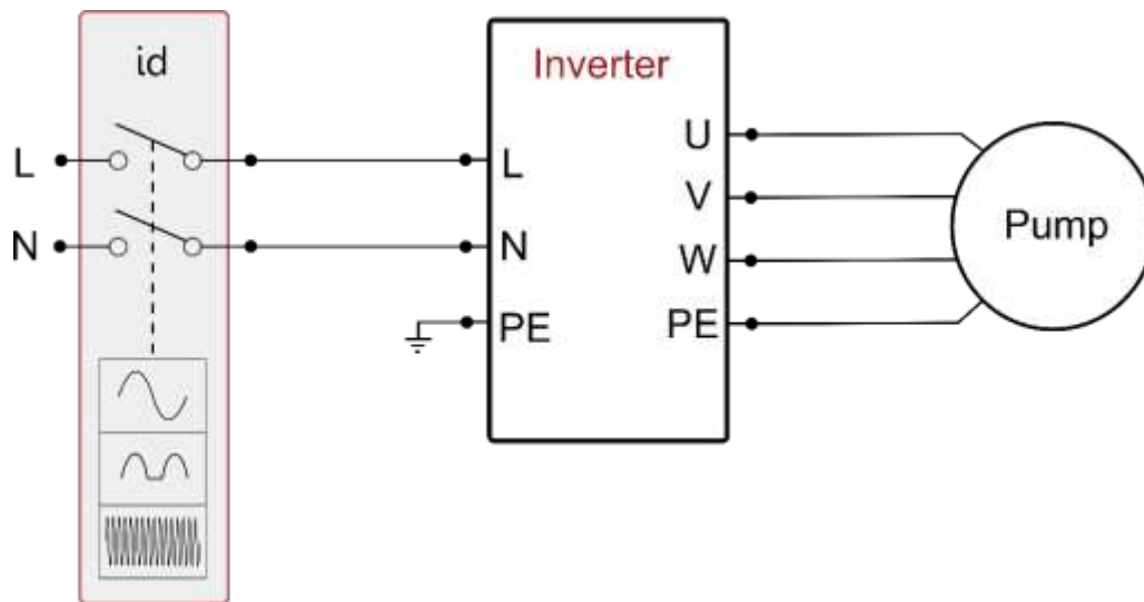
Σχήμα 3a: Παράδειγμα εγκατάστασης με μονοφασική τροφοδοσία
