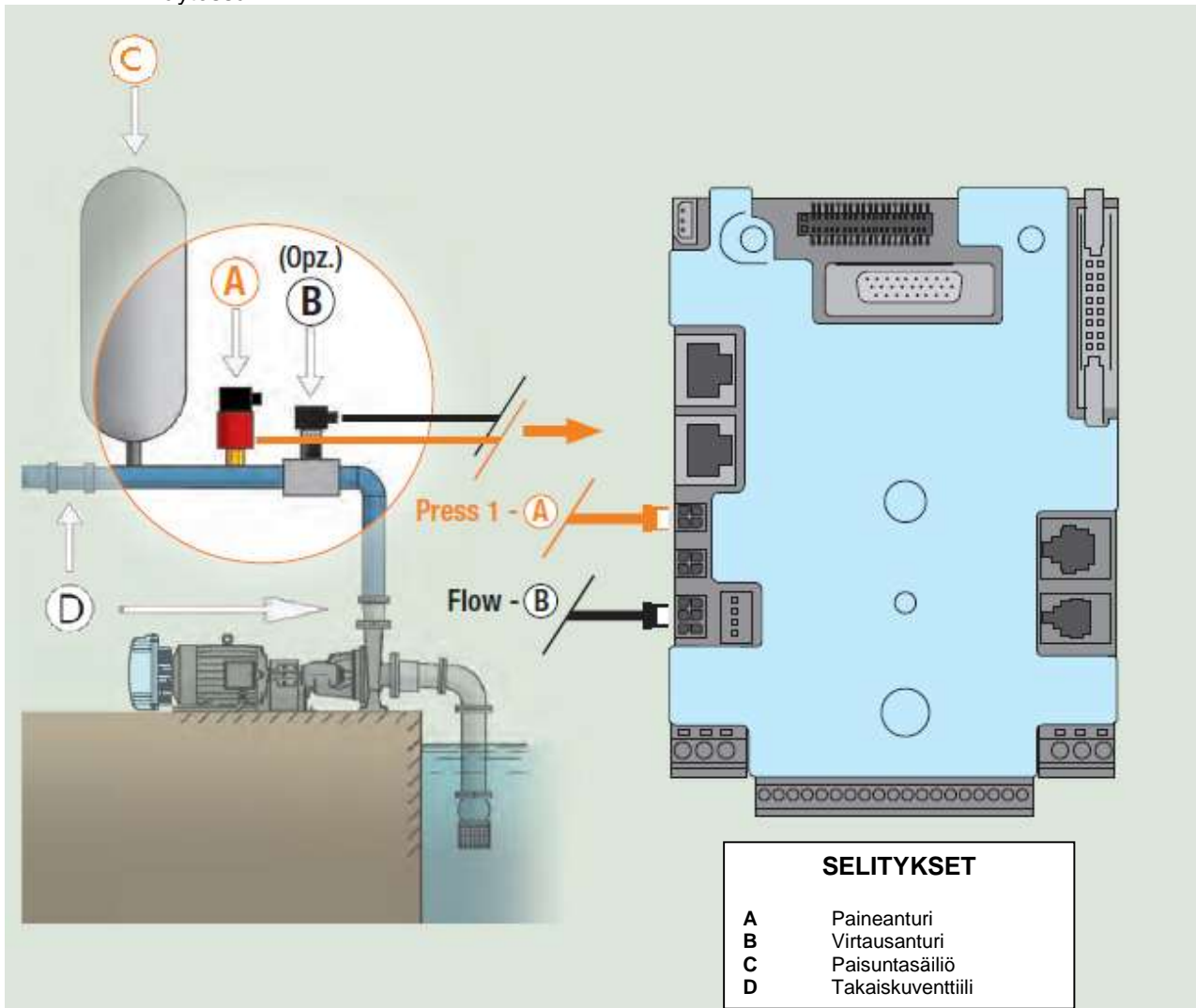
Kuva 7: Hydrauliasennus
