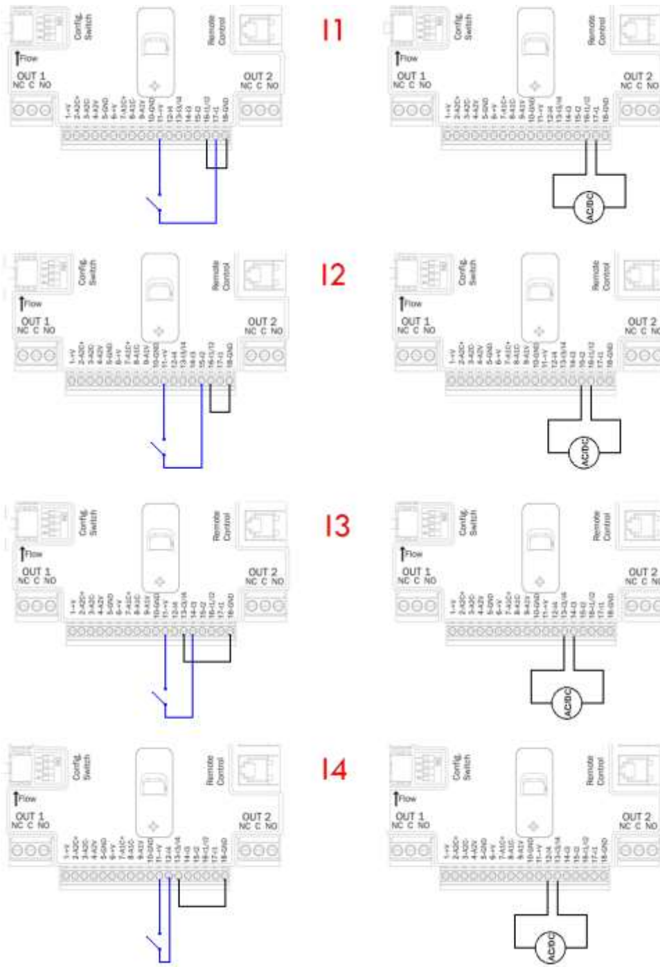
Рисунок 12: Пример соединения входов
