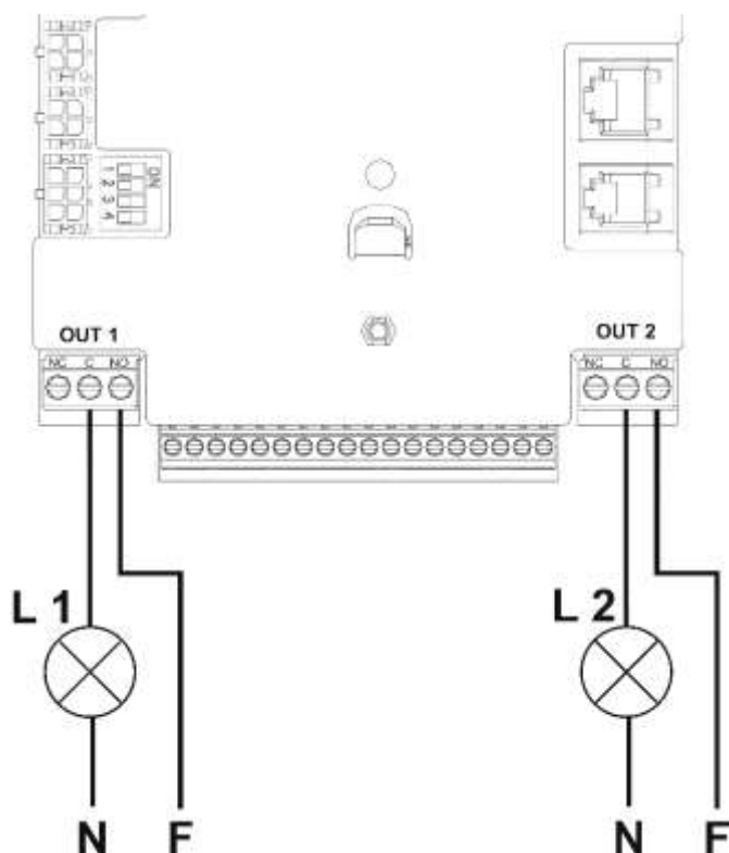
Рисунок 11: Пример соединений выходов
