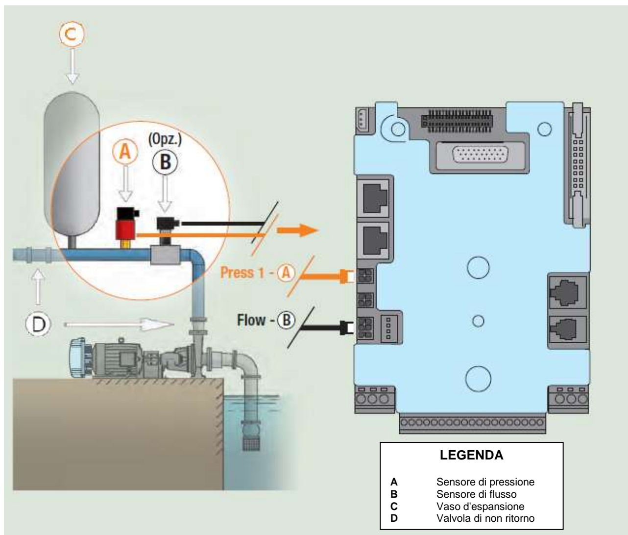
Figura 7: Installazione Idraulica
