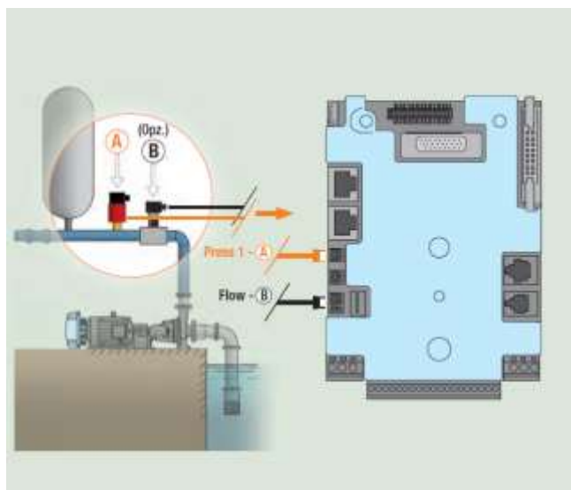
Figura 8: Connessioni sensori
