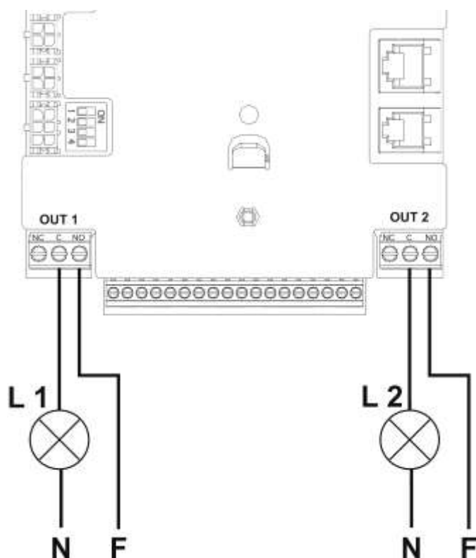
Kuva 11: Esimerkki lähtöjen liittännästä
