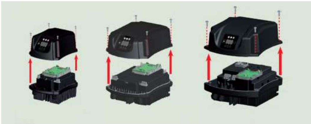
Obrázek 2: Sejmutí krytu pro přístup k připojení
