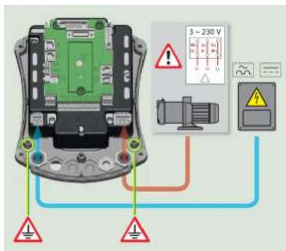
Obrázek 6: Zapojení čerpadla MCE 22/P – MCE 15/P – MCE 11/P
