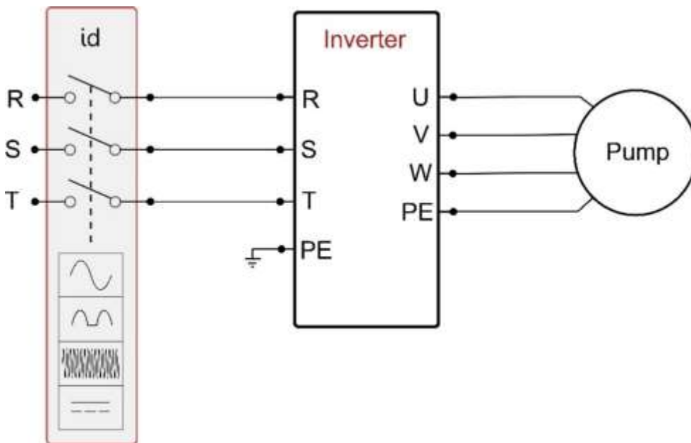
Рисунок 4b: Пример установки при трехфазном питании
