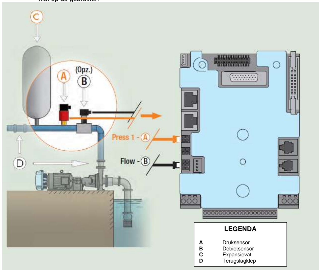
Afbeelding 7: Hydraulische installatie
