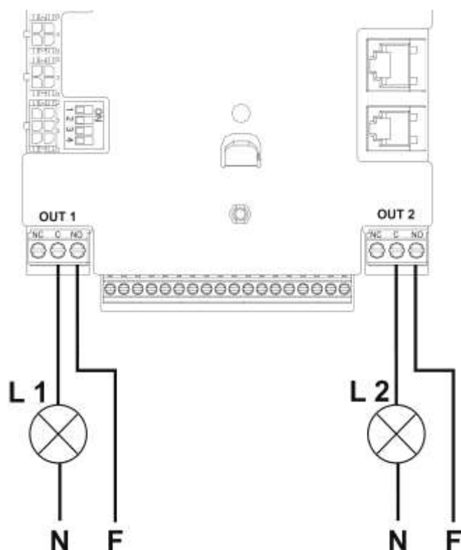
Σχήμα 9: Παράδειγμα σύνδεσης των εξόδων
