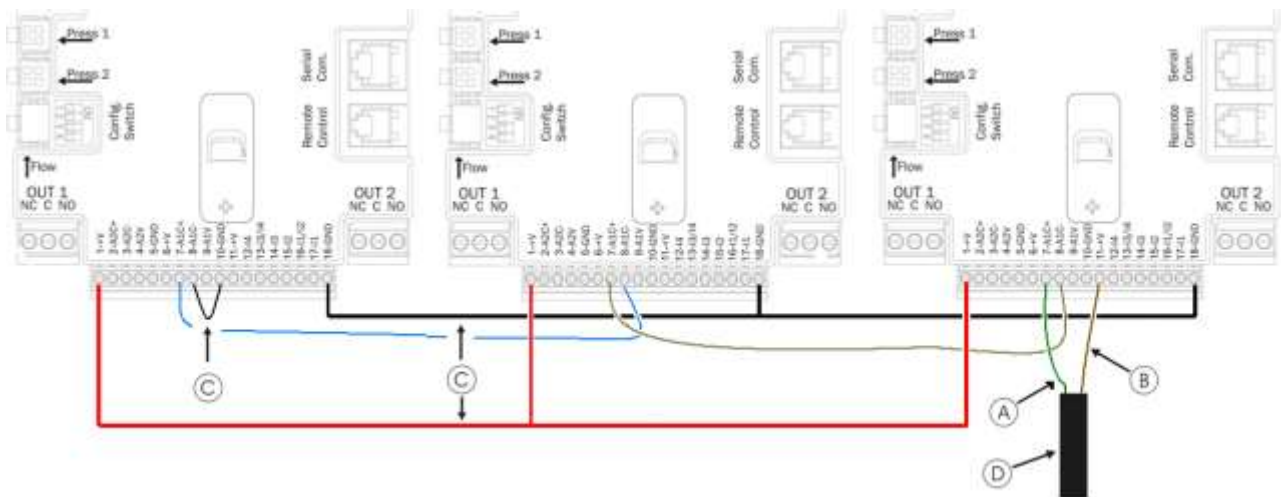
Fig. 10: Anslutning av trycksensor 4 - 20 mA i ett system med flera invertrar
