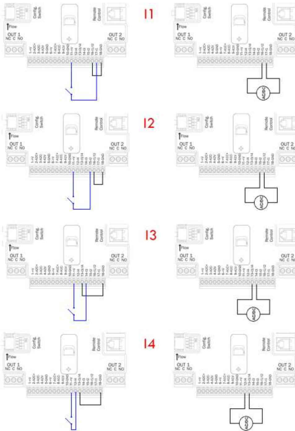
Afbeelding 12: Voorbeeld van aansluiting van de ingangen
