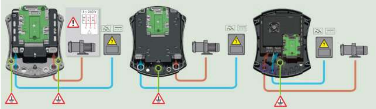
Şekil 5: Elektrik bağlantıları
