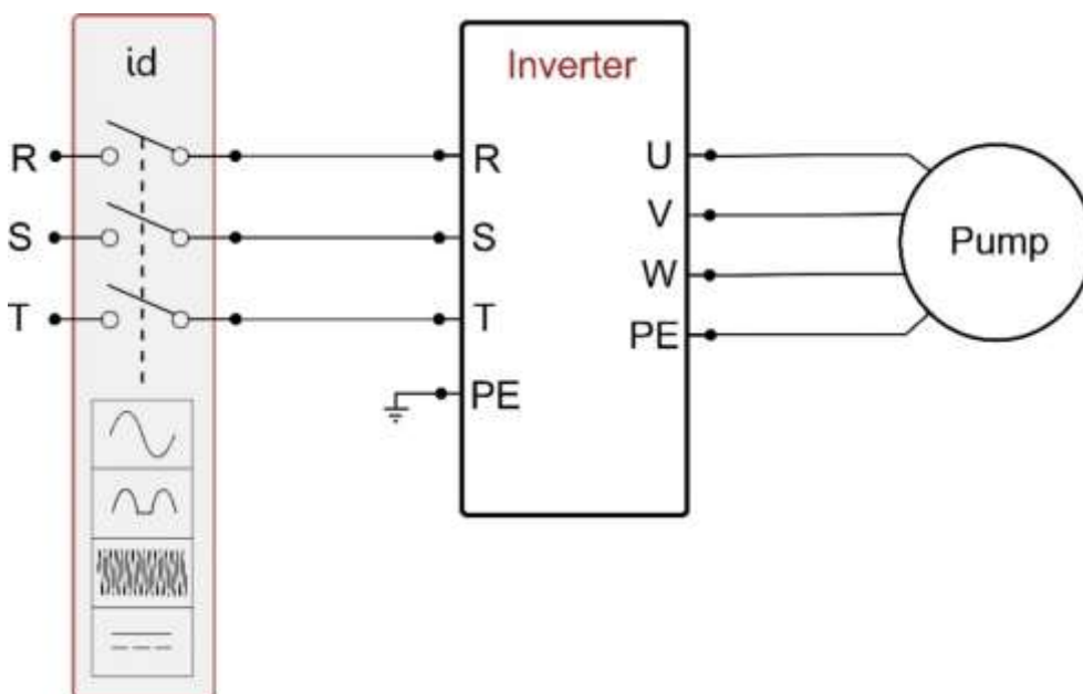
Abbildung 4b: Beispiel einer Installation mit Dreiphasenversorgung
