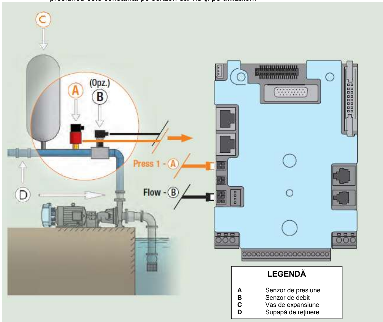
Figura 7: Instalația hidraulică
