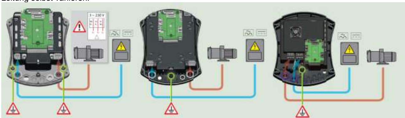
Abbildung 5: Elektrische Anschlüsse
