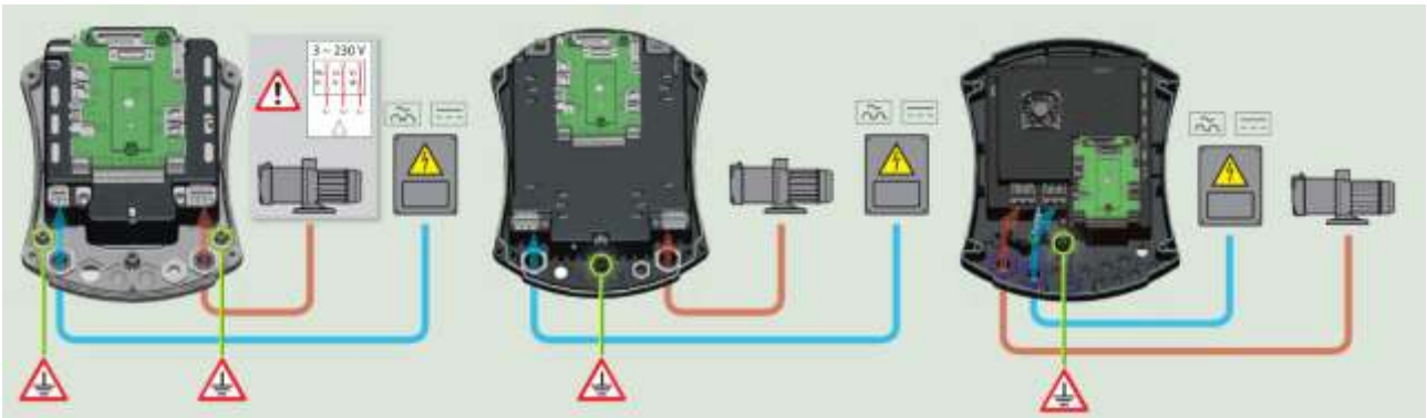
Figura 5: Conexiones eléctricas
