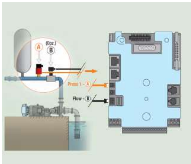
Σχήμα 8: Συνδέσεις αισθητήρων
