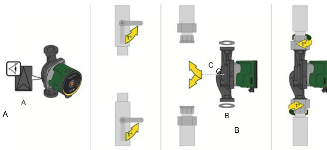
Rysunek 2: Montaż modelu EVOSTA2 lub EVOSTA3
