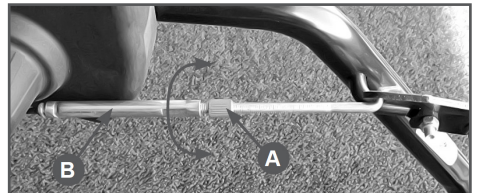
Рис.24 Регулировка троса привода хода
