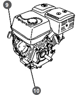
Рис.12 (А) Основные узлы и органы управления двигателем ST656
