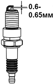
Рис.17 Свеча зажигания
