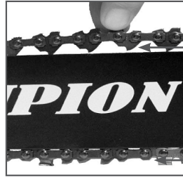
Рис.8 Правильное натяжение цепи
