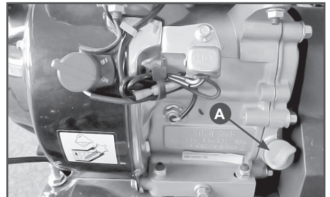
Рис.10 Заправка маслом нового двигателя
