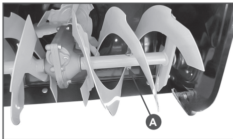
Рис.16 Замена срезного болта шнека
