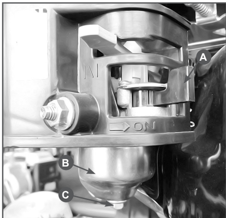
Рис.18 Удаление топлива из бака
