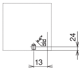
Место подсоединения дренажной трубки
