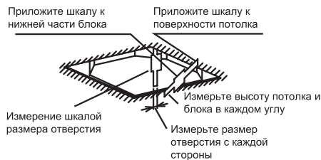
Трафарет для установки
