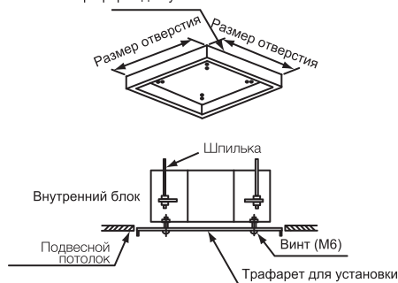
Трафарет для установки
